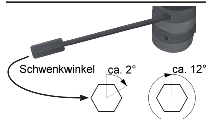
Einstellwerkzeug eingesteckt
