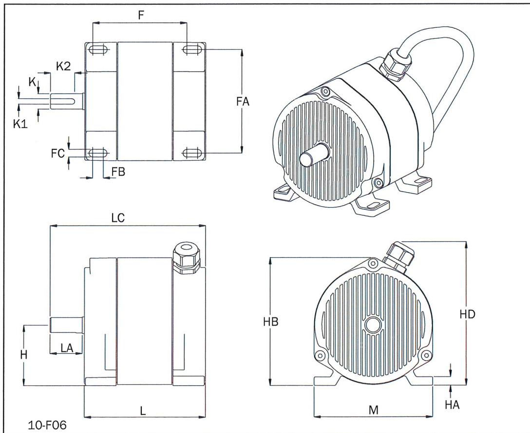
Abb. 7 Abmessungen - Motor
